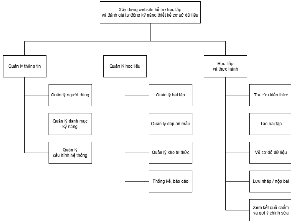
Hình 3.2 Sơ đồ phân cấp chức năng của hệ thống
