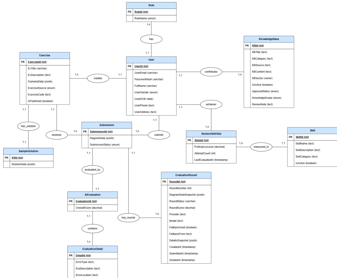
Hình 3.1 Mô hình dữ liệu của ứng dụng
