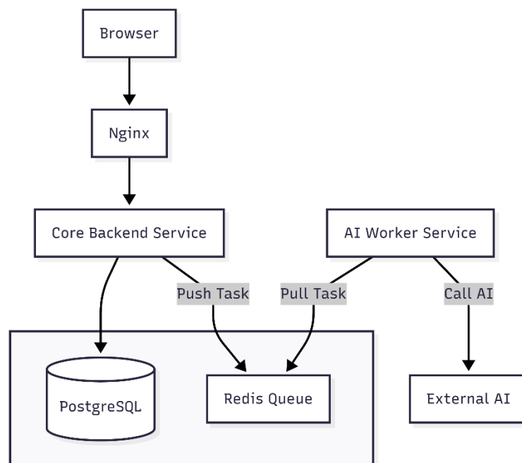
Hình 3.15 Kiến trúc chung của hệ thống
