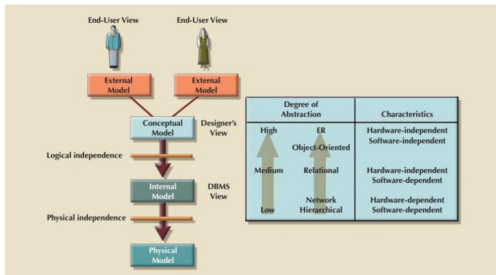
Hình 2.3 Các mức độ của thiết kế CSDL [2]
